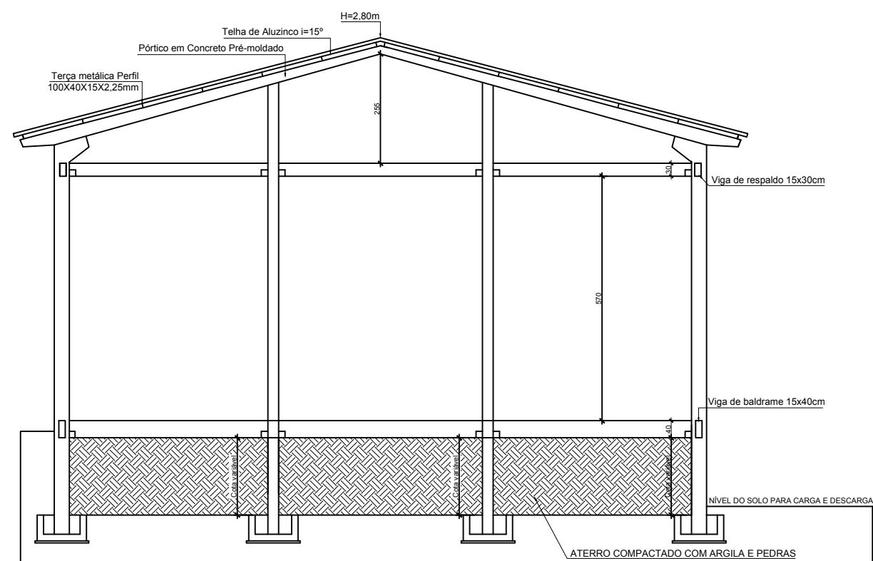
CORTE (Vista frontal - ampliação)
