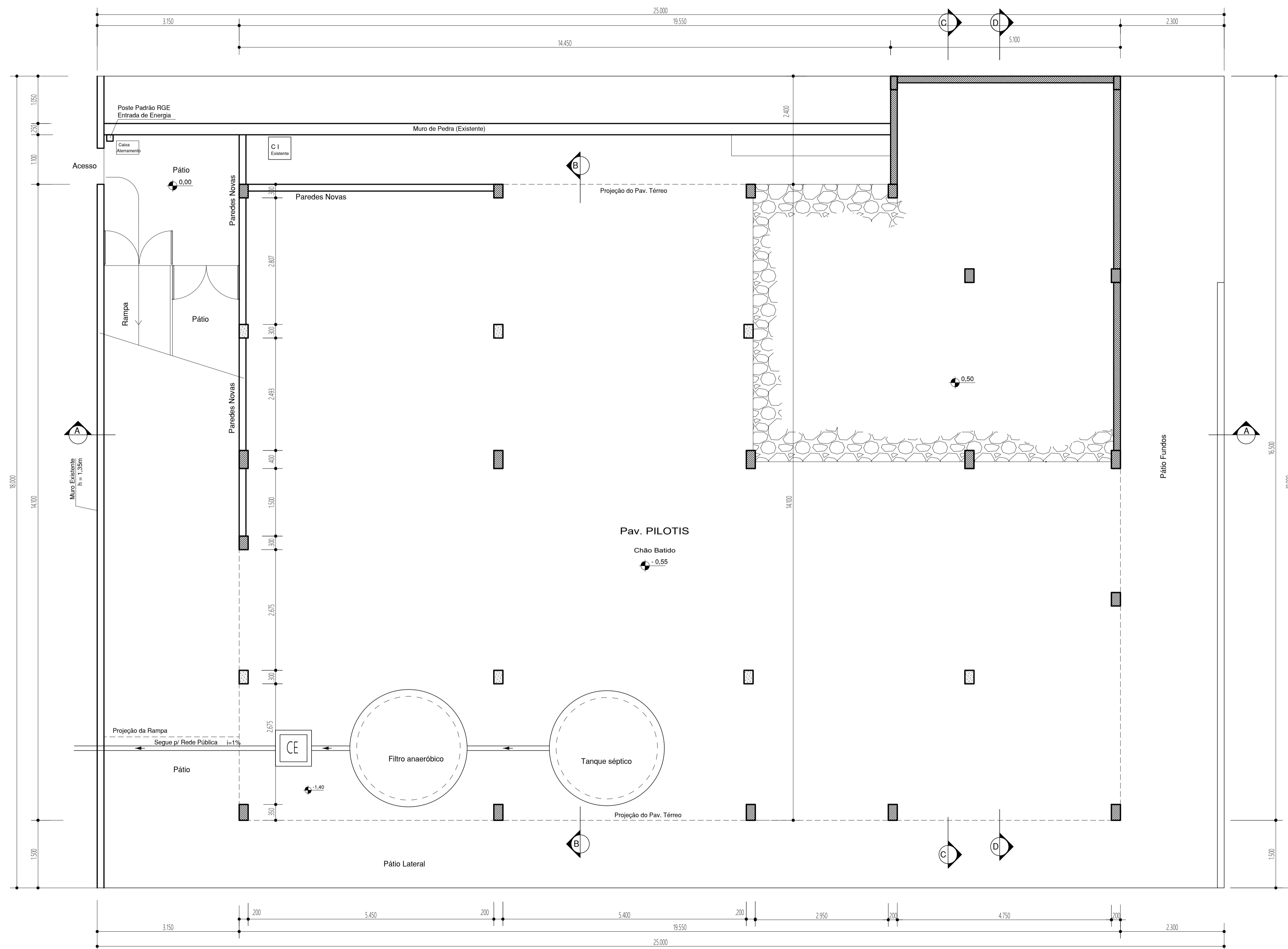
Planta Baixa Pilotis 1:50 Área=287,89 m 2
