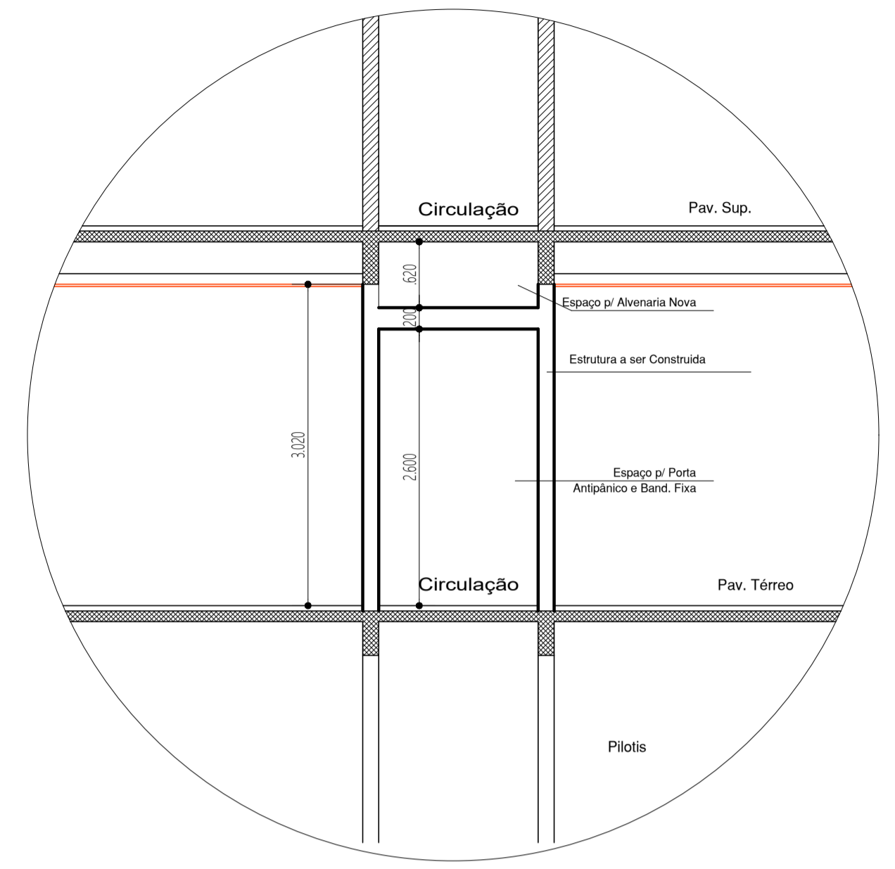
DET. 01: PILATERES E VERGA TRAVAMENTO
