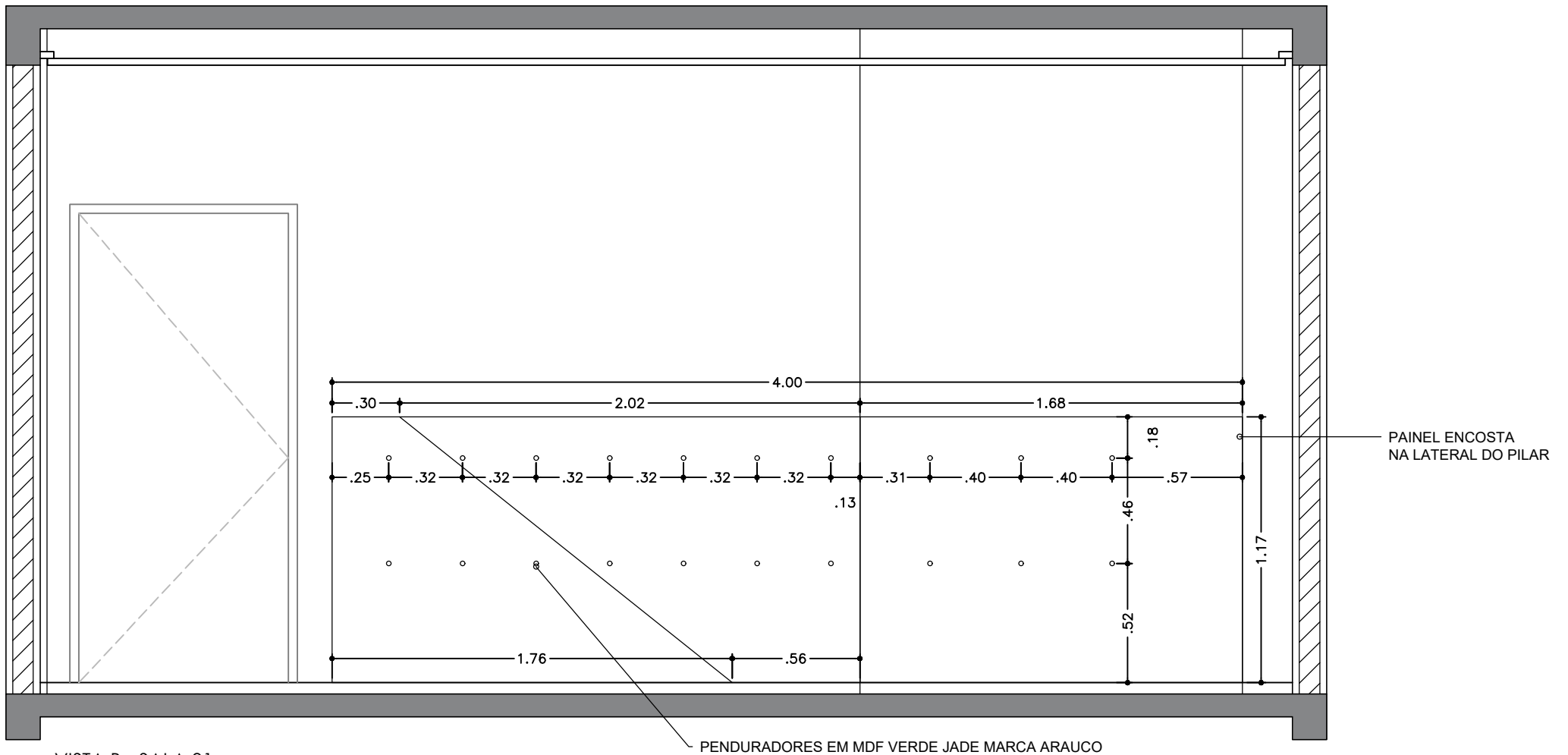
5 VISTA B - SALA 01 ESC. 1:25
