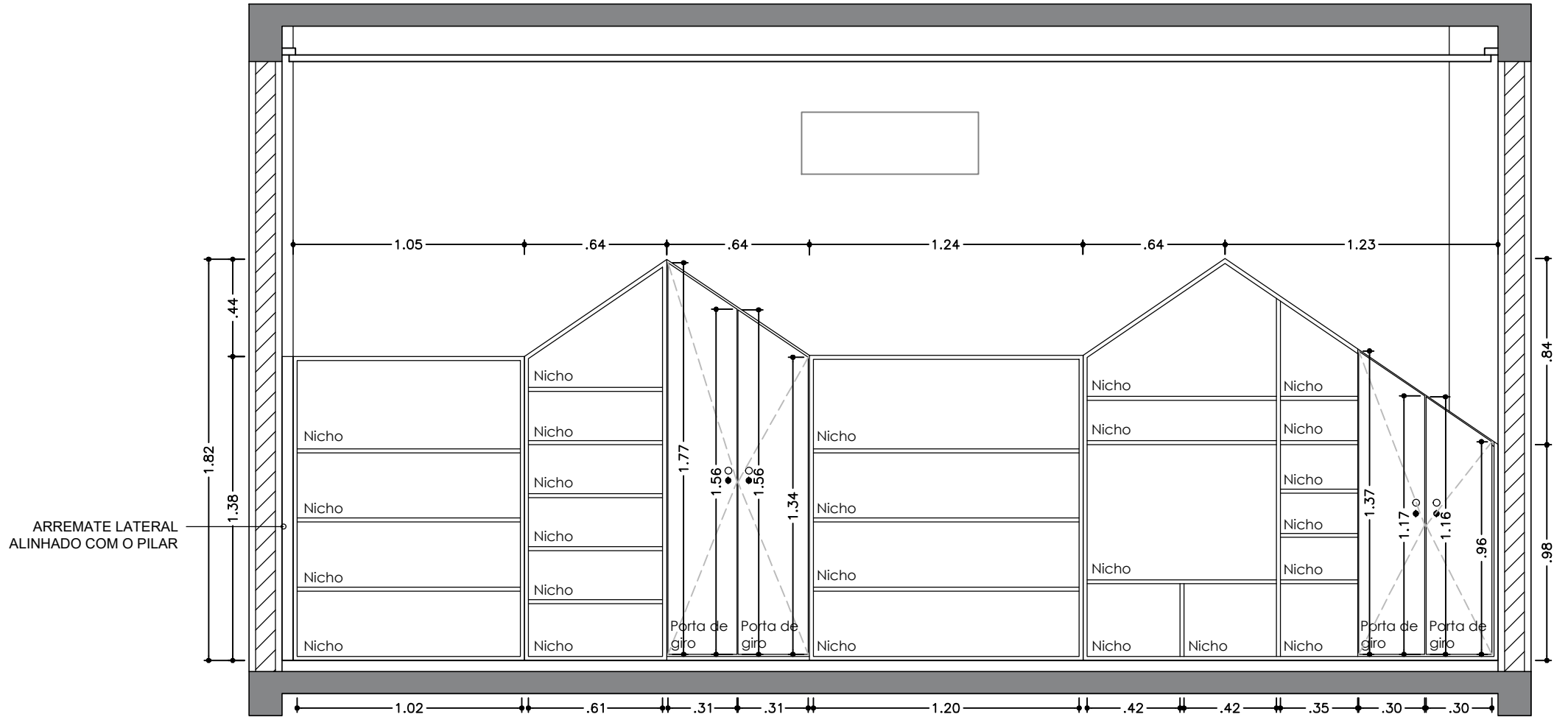
2 VISTA A - SALA 03 ESC. 1:25
