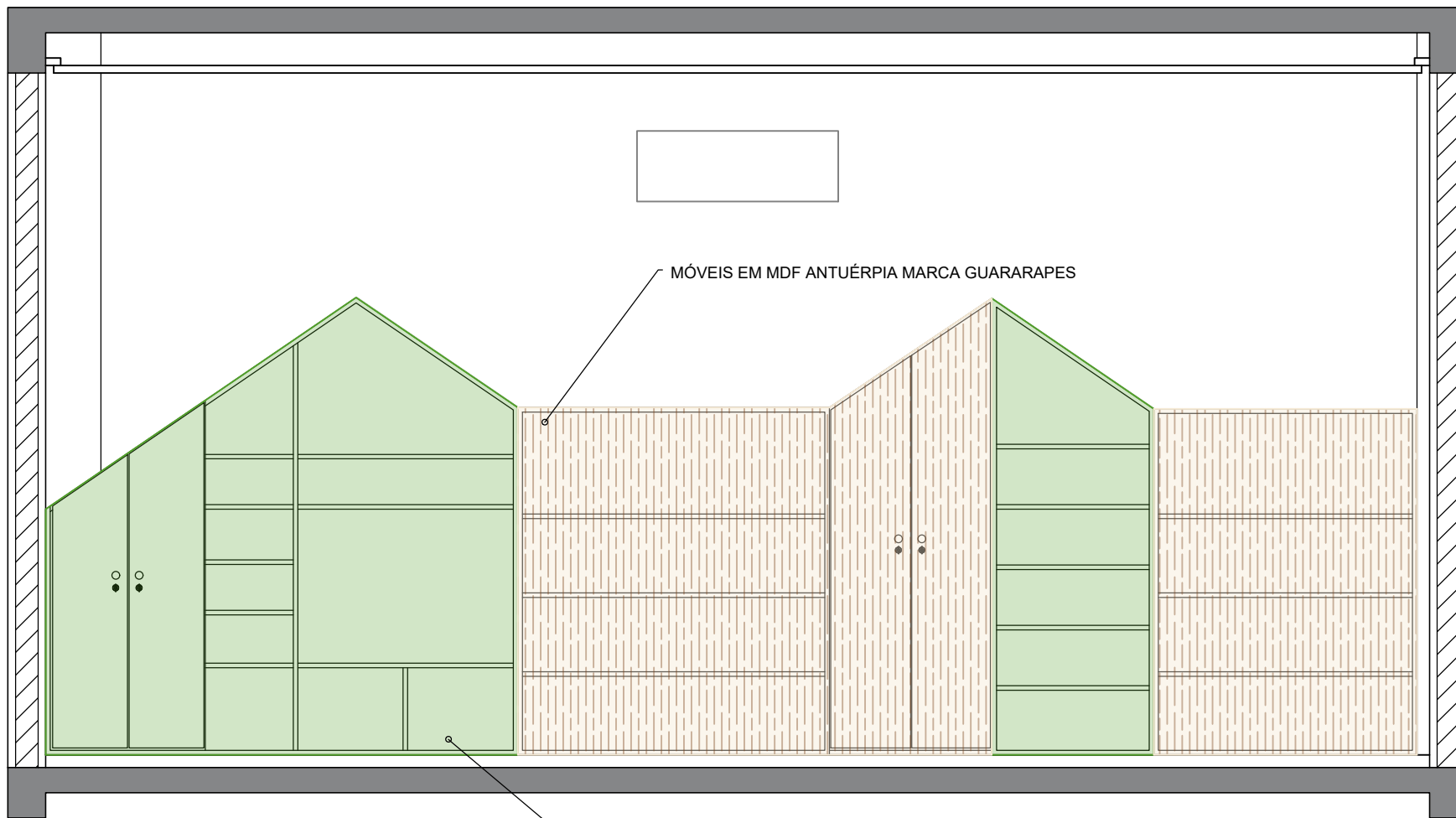
4 VISTA A - CORES - SALA 01 ESC. 1:25
