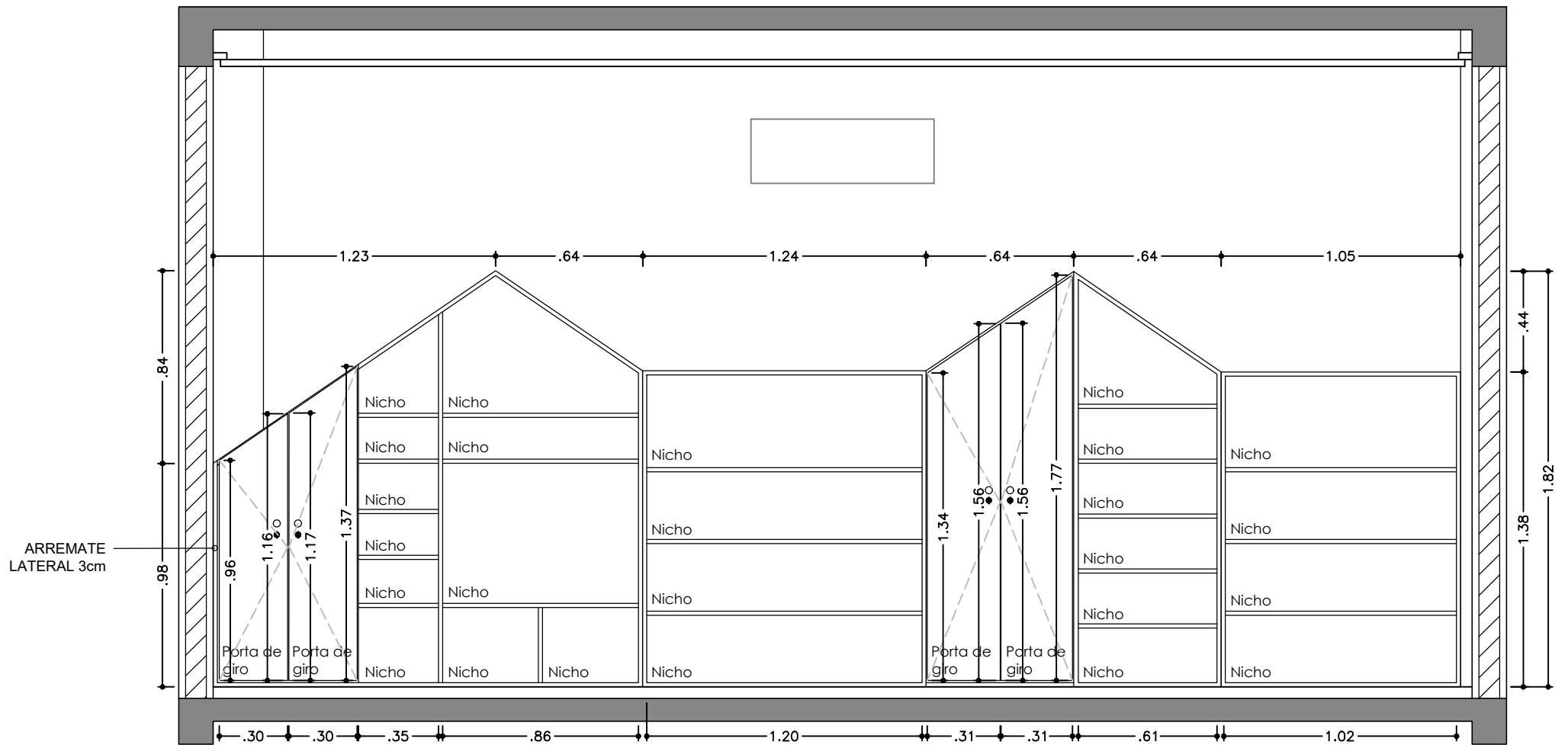
2 VISTA A - SALA 01 ESC. 1:25
