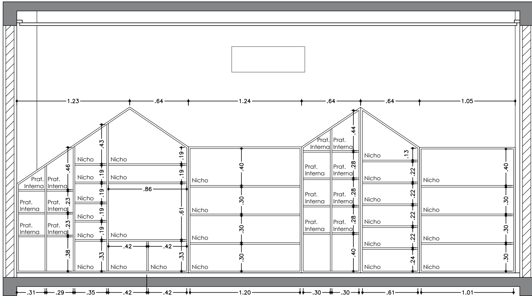
3 VISTA A - INTERNA - SALA 01 ESC. 1:25
