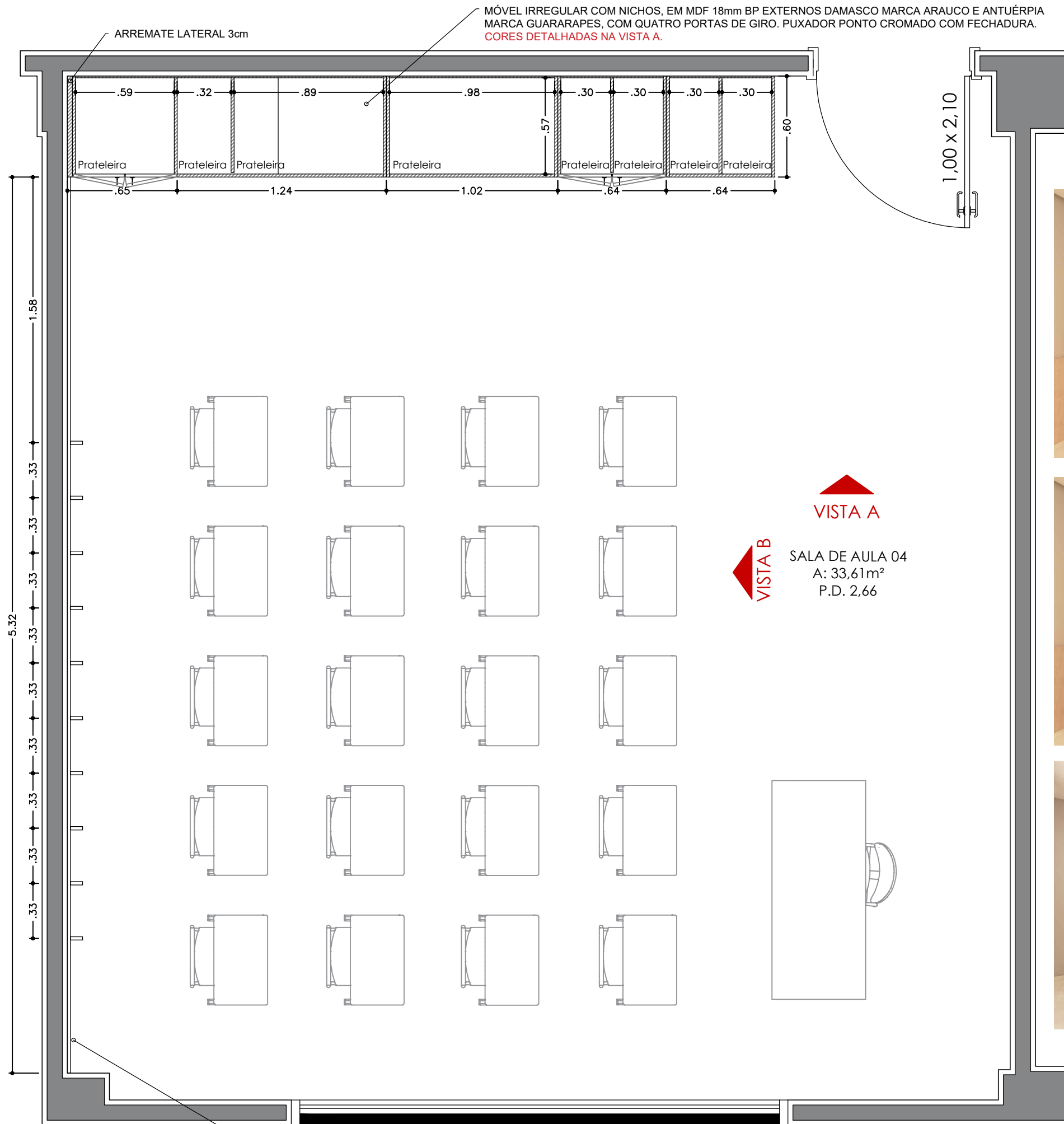
1 PLANTA BAIXA - SALA 04 ESC. 1:25
