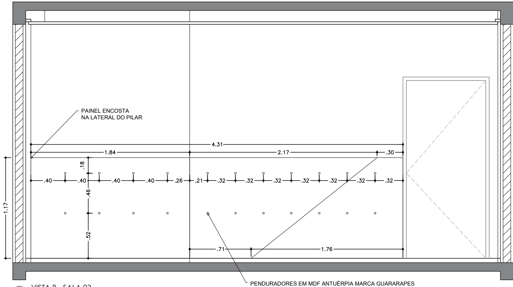
5 VISTA B - SALA 03 ESC. 1:25
