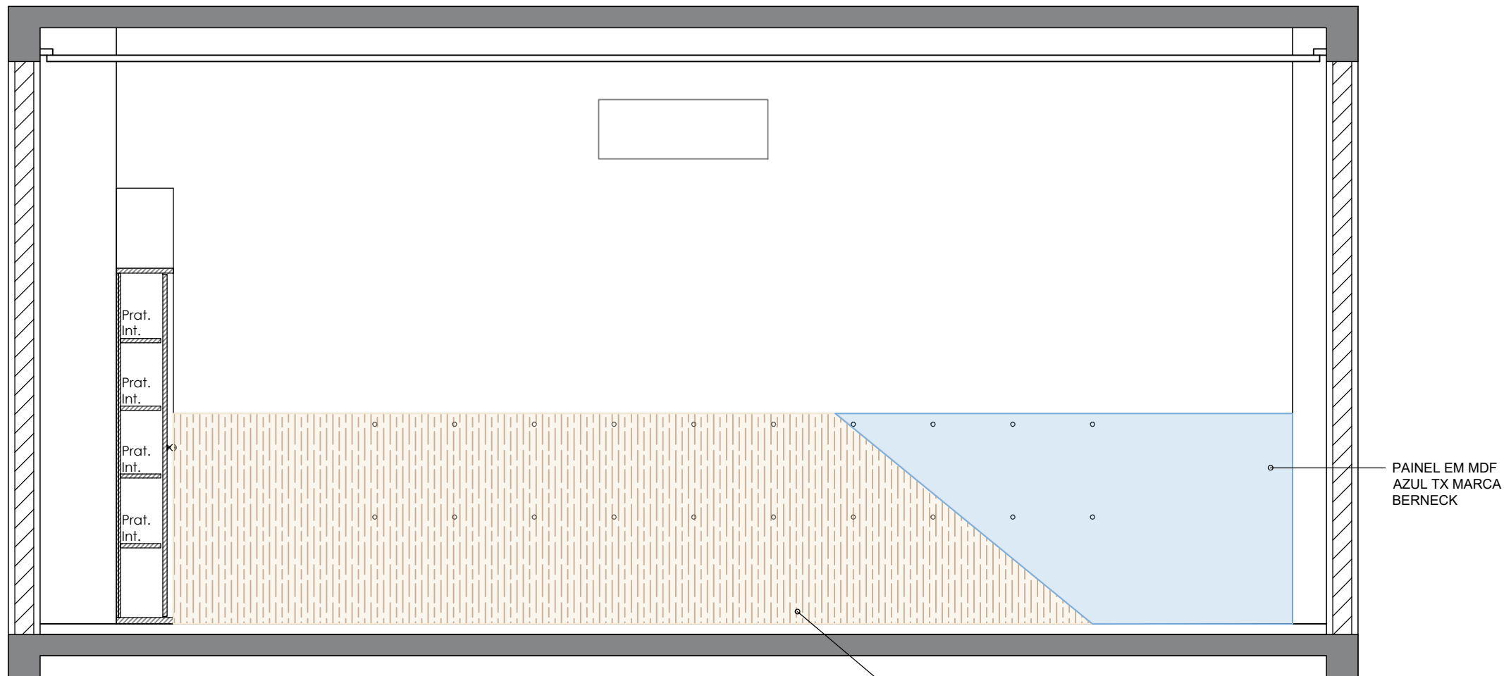
6 VISTA B - CORES - SALA 02 ESC. 1:25
