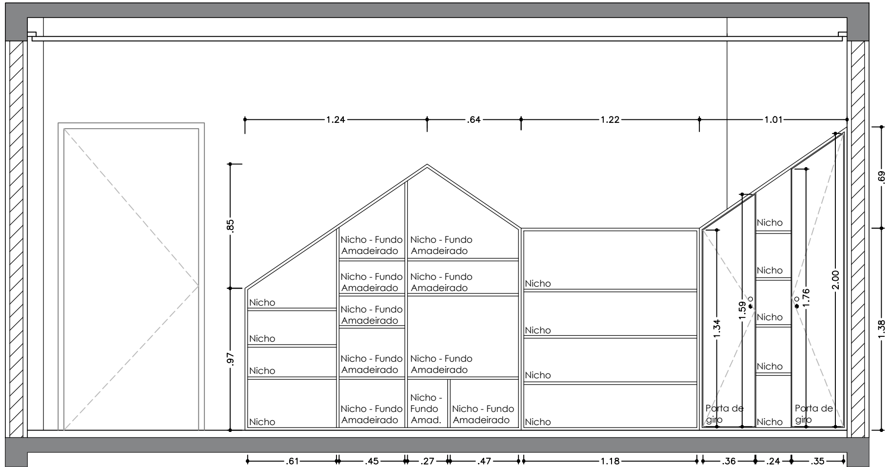
2 VISTA A - SALA 02 ESC. 1:25
