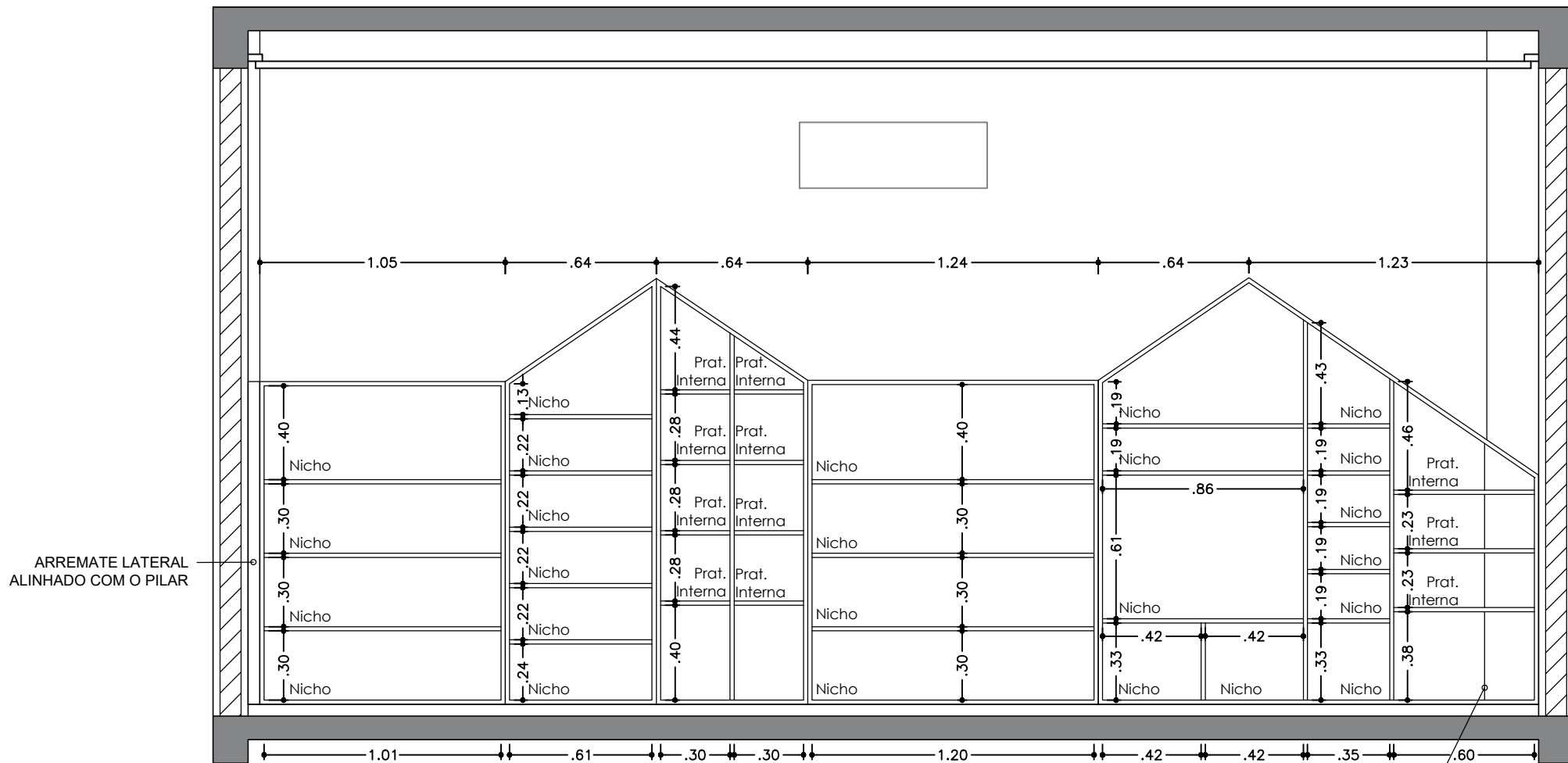
3 VISTA A - INTERNA - SALA 03 ESC. 1:25
