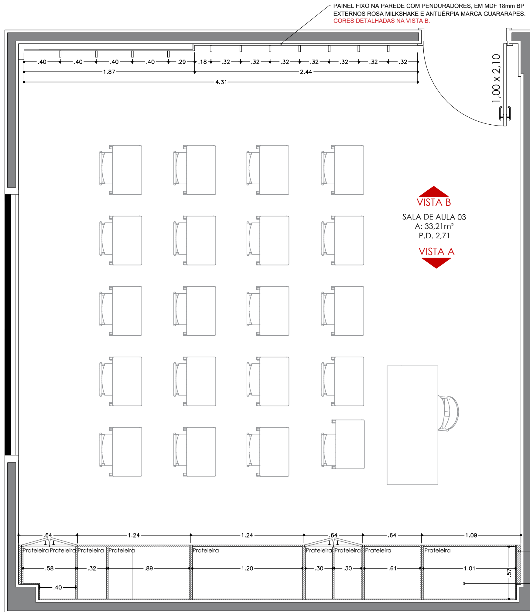
1 PLANTA BAIXA - SALA 03 ESC. 1:25
