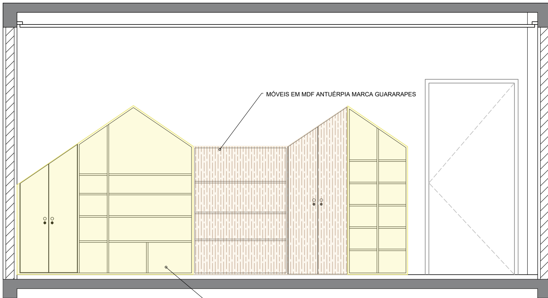
4 VISTA A - CORES - SALA 04 ESC. 1:25
