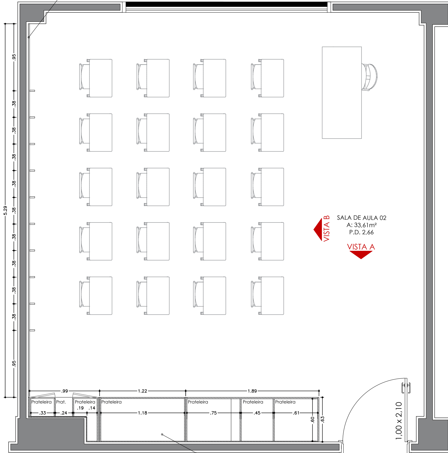
1 PLANTA BAIXA - SALA 02 ESC. 1:25
