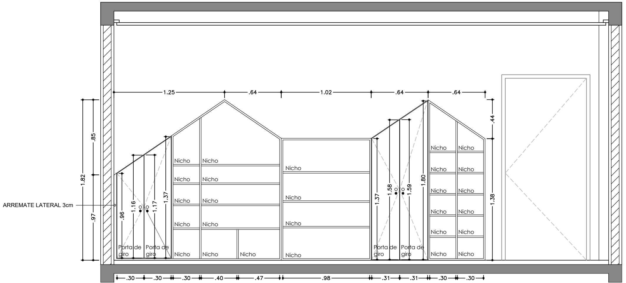
2 VISTA A - SALA 04 ESC. 1:25
