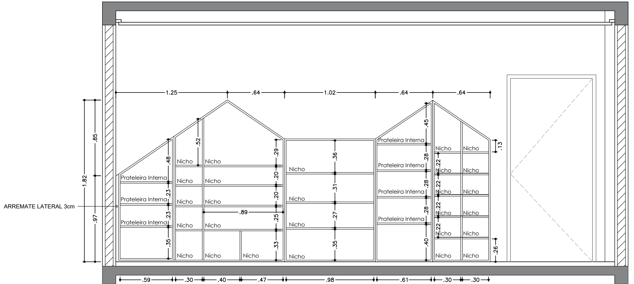
3 VISTA A - INTERNA - SALA 04 ESC. 1:25
